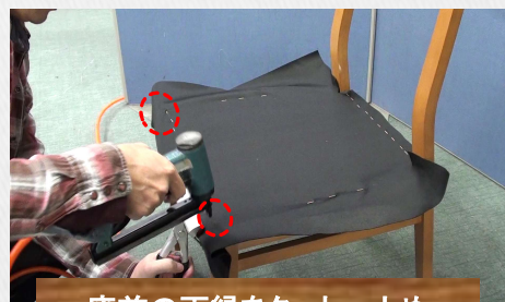
座前の両縁をタッカー止め
